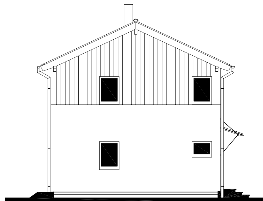
POHLED BOČNÍ /PRAVÝ/
